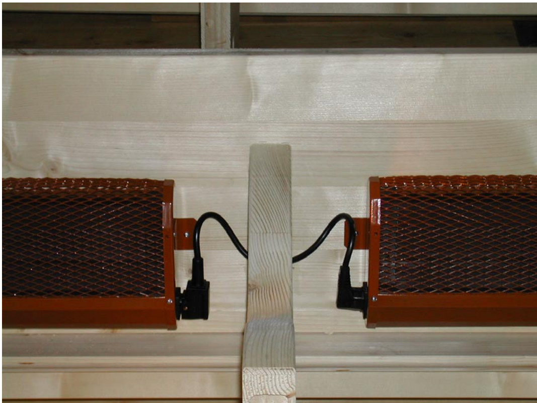
6. Montage: Verbindungsleitung
